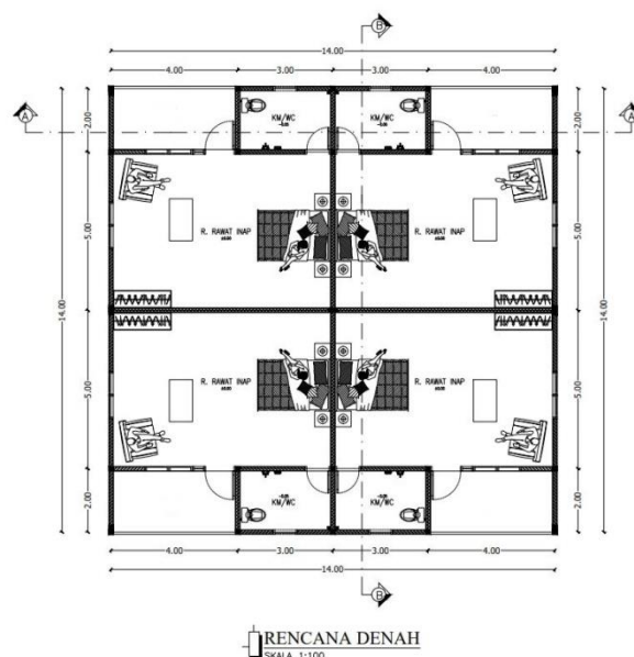
Het gedeeltelijk aanwezige gebouw dat als basis dient voor de isolatiekamers
